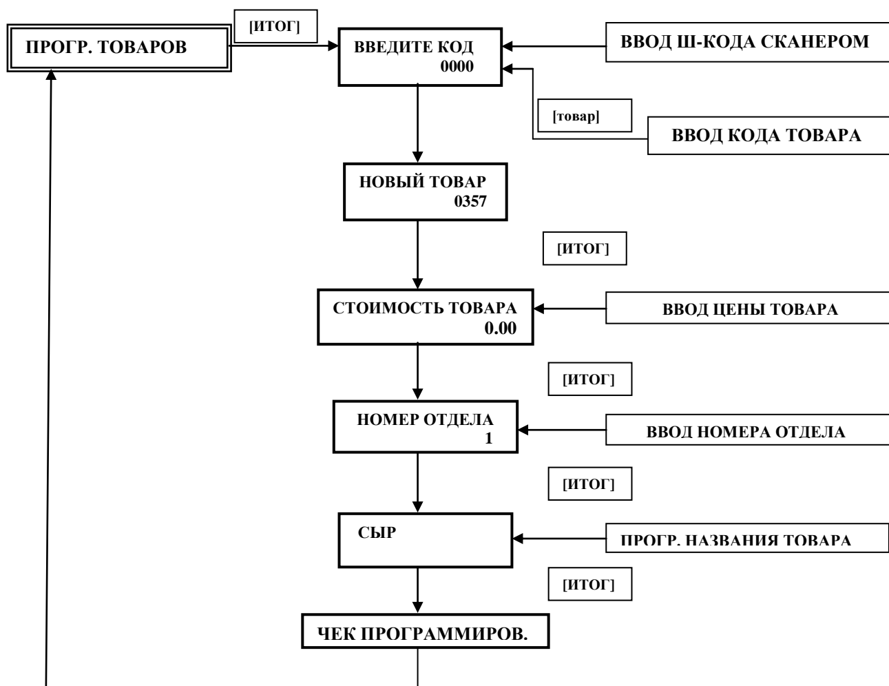
Рис.10.5. Структурная схема раздела «Программирование товаров».
