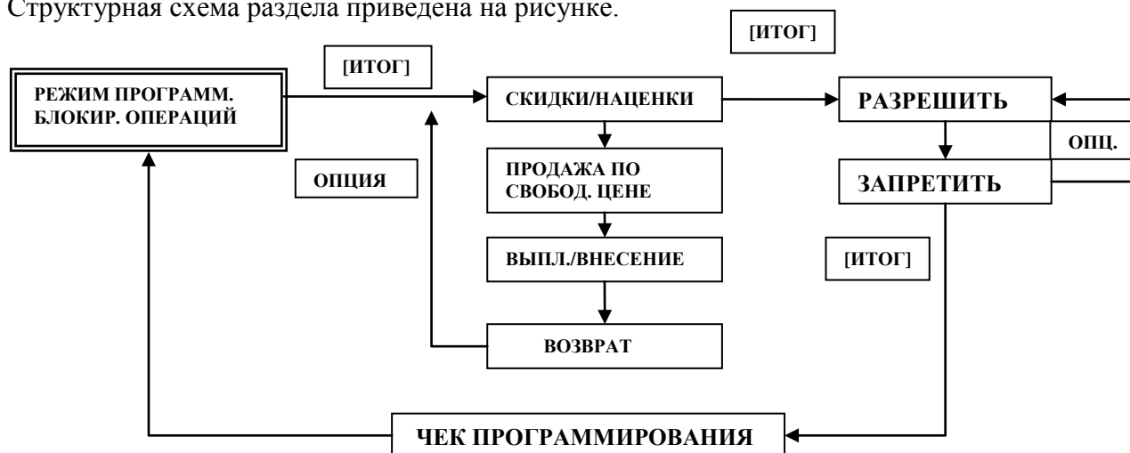
Рис.10.6. Структурная схема раздела «Блокировка операций».
