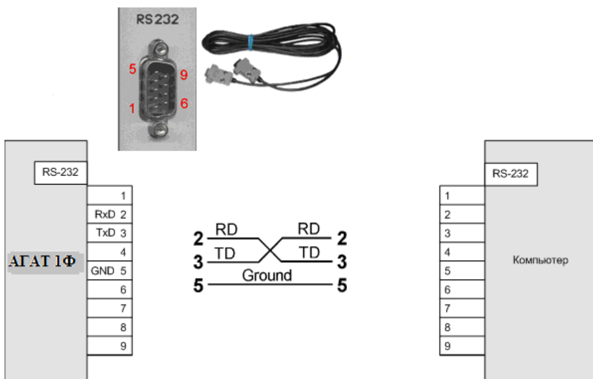
Рис. П.1.1. «Нуль-модемная» связь ККТ с компьютером.
